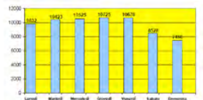
GRAFICO - Transito giornaliero dei veicoli
